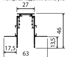
Шинопровод ГКЛ 12,5 мм
