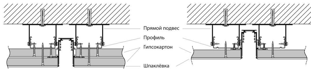
Два слоя гипсокартона
