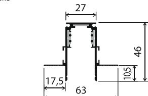
Шинопровод ГКЛ 9,5 мм
